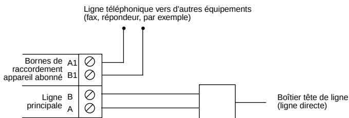
Figure 17. Raccordement de la ligne téléphonique
