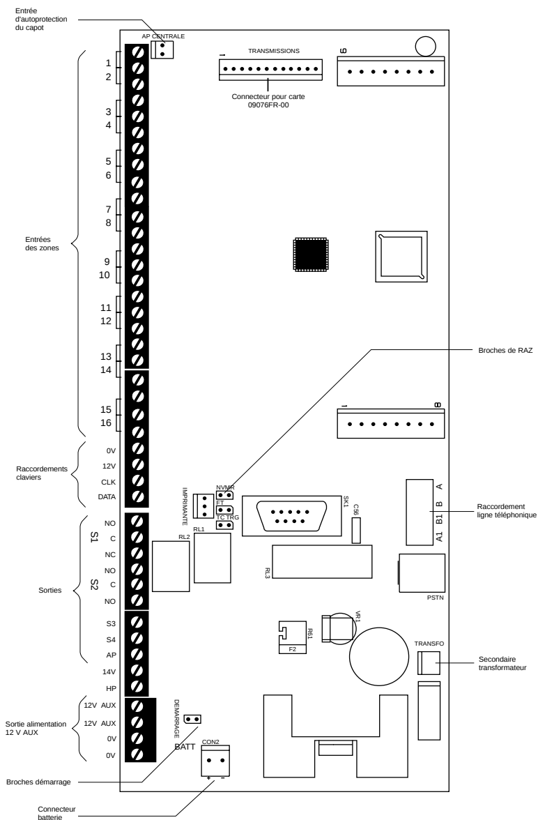
Figure 3. Circuit imprimé de la centrale
