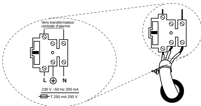
Figure 7. Raccordement secteur
