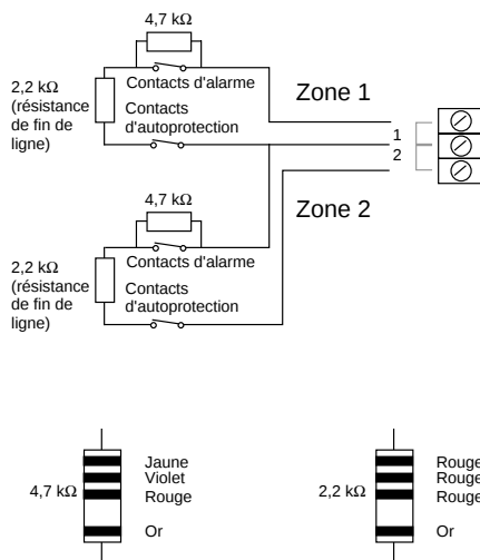
Figure 11. Raccordement de zones filaires supervisées
