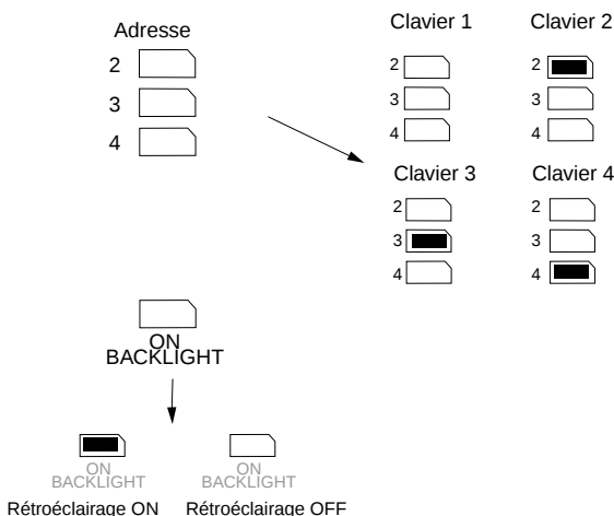
Figure 8. Adressage des claviers
