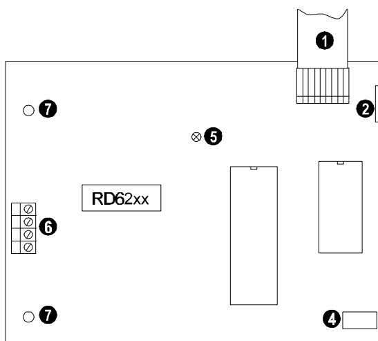
Figure 1: Schéma du RD6202S33
