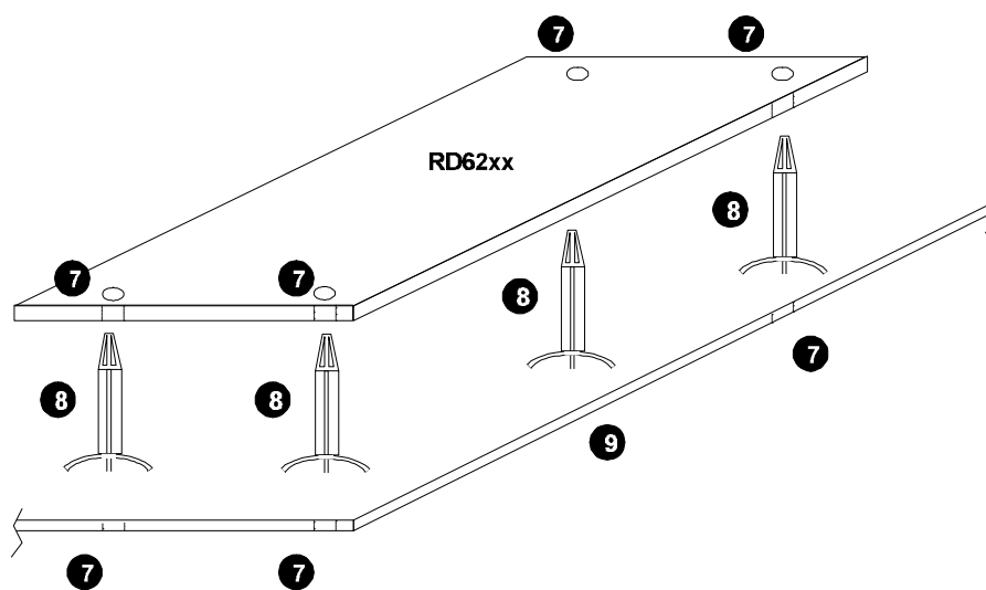
Figure 3: Fixation du RD6202S33
