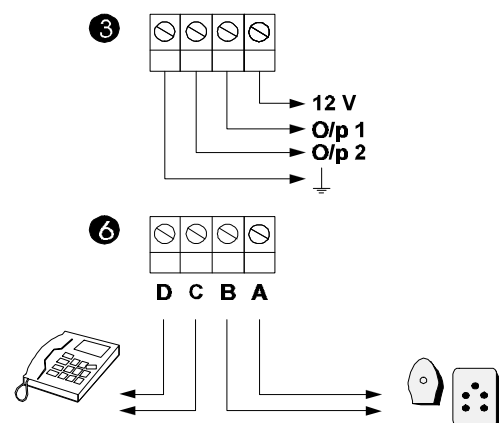
Figure 2: Connexions du RD6202S33
