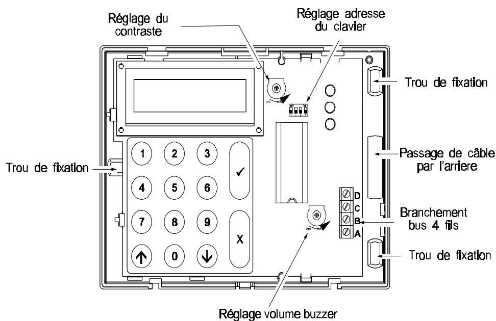
Figure 15. Clavier CD3008/9S33
