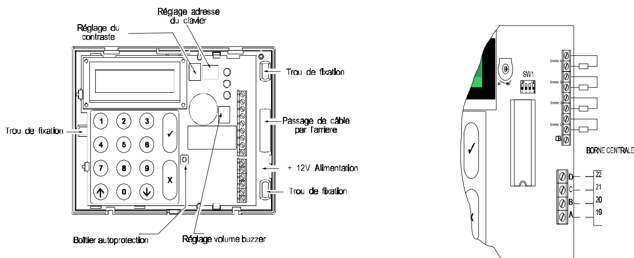
Figure 16. Clavier CD3048/9S33
