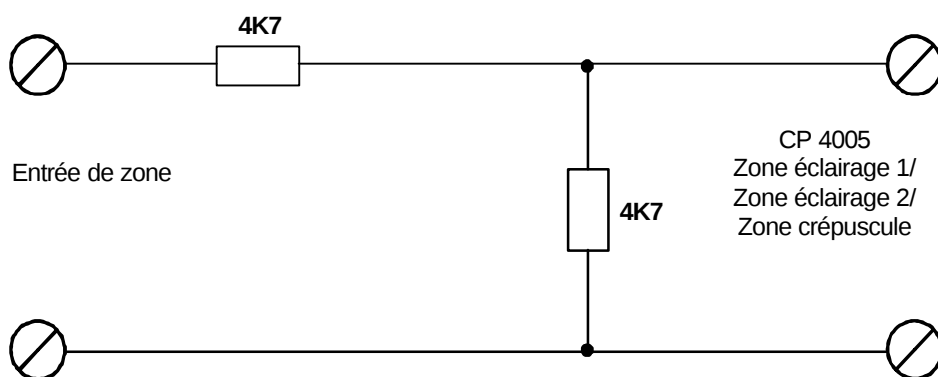
Figure 21. Câblage d'une carte Nitewatch CP4005
