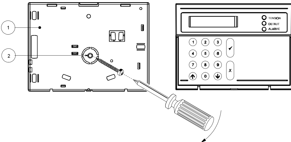
Figure 18. Autoprotection à l'arrachement des claviers
